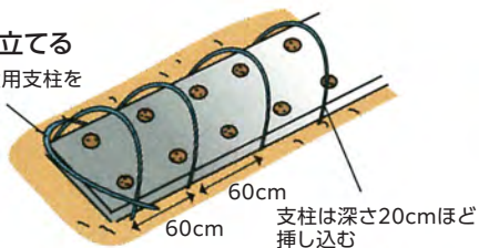
図 トンネルの作り方
